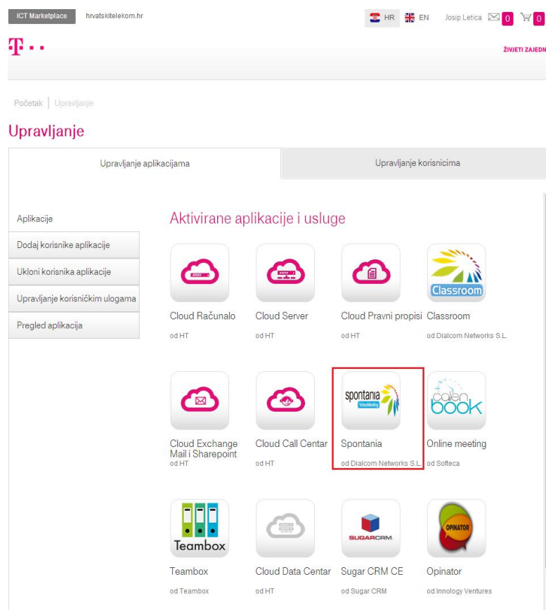
Slika 5. Prikaz aplikacije/a
