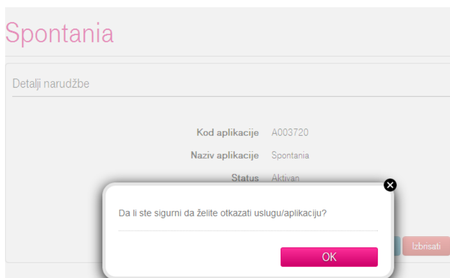
Slika 10. Pop-up potvrda
