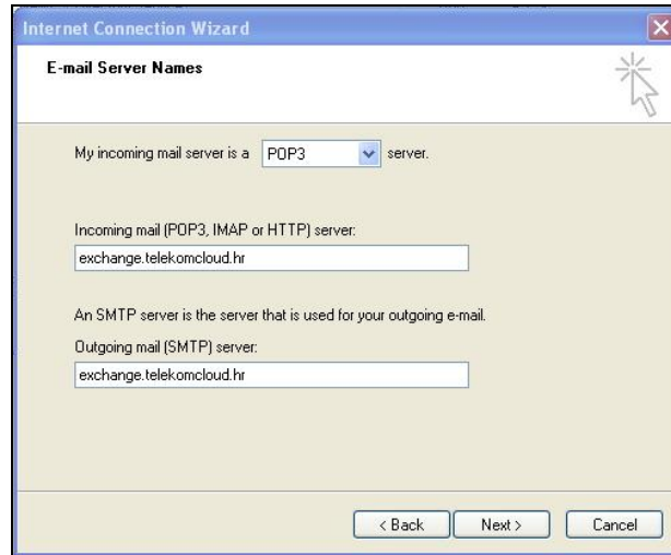
Slika 3. Konfiguracija poslužitelja
